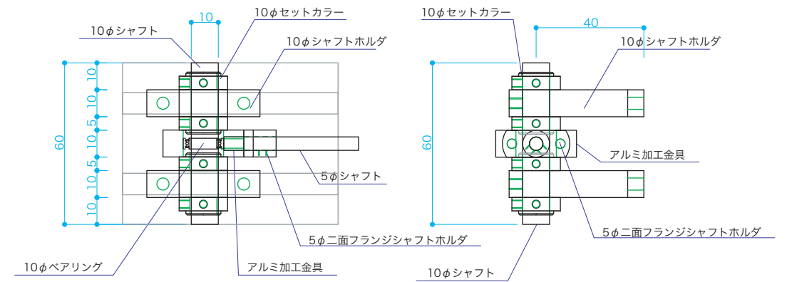
磁力カッター 鉄片回転部 S=1/2
