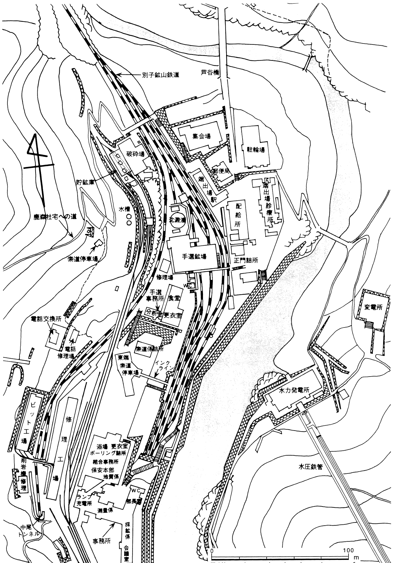
図5 昭和初期の端出場（図3枠線を拡大） 別子銅山記念館所有資料 1/1,200端出付近地形図（昭和23年3月15日）及び井上氏からの聞き取りをもとに作成
