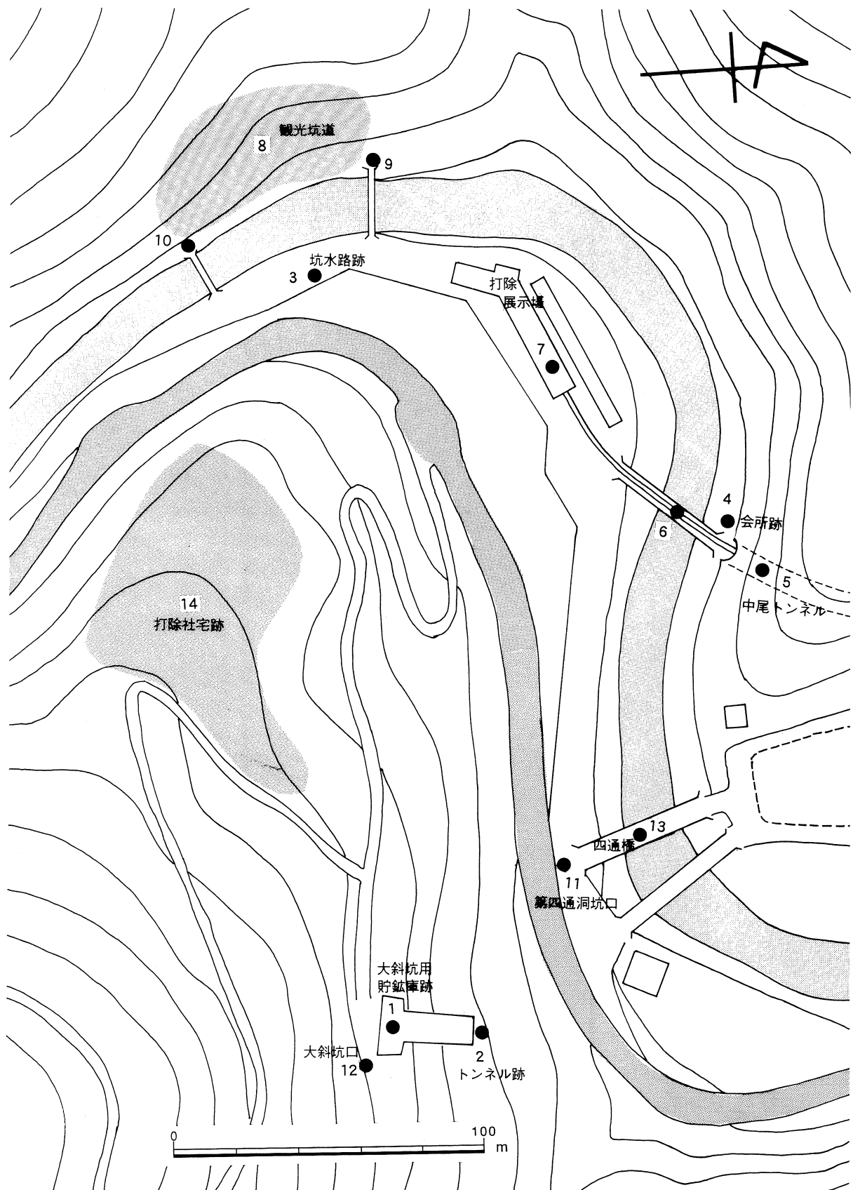
図6 現在の打除（図3 枠線を拡大） 国土地理院発行1/5,000森林基本図（IV-GD65）より作成
