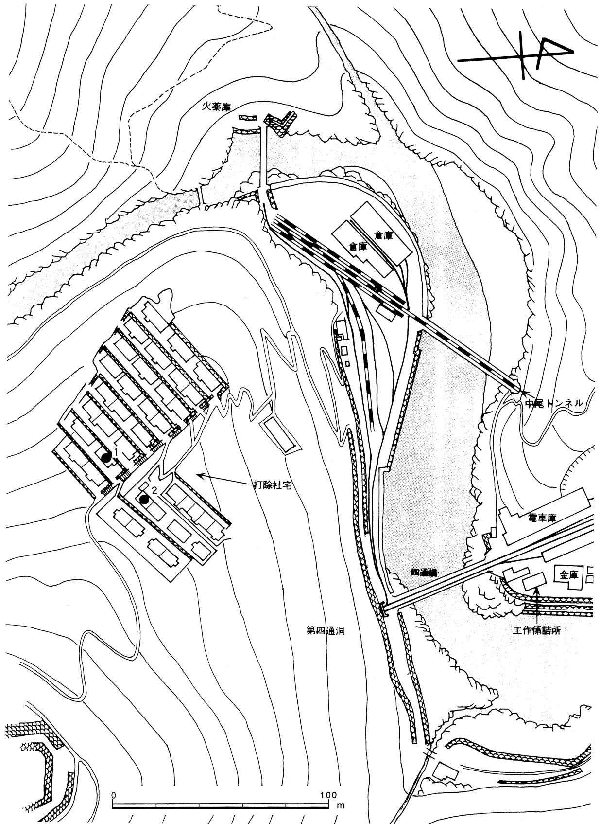
図7 昭和初期の打除（図3 枠線を拡大） 別子銅山記念館所有資料 1/1,200端出場付近地形図（昭和23年3月15日）及び井上氏からの聞き取りをもとに作成
