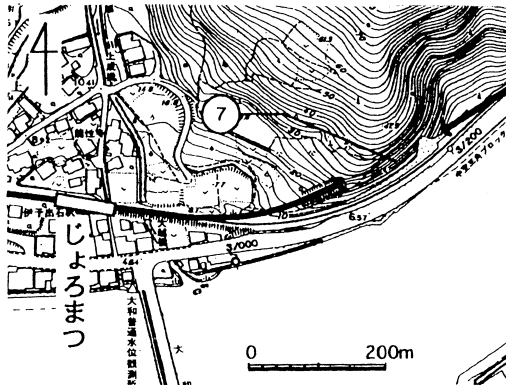
図5-C 愛媛鉄道路線図（旧大越トンネル付近） 肱川流域平面図（1/2,500）No.6より作成
