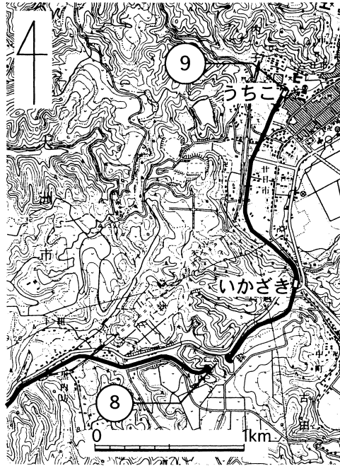
図5-E 愛媛鉄道路線図(旧二本松トンネル～旧内子駅付近) 国土地理院発行1/25,000地形図「内子」より作成
