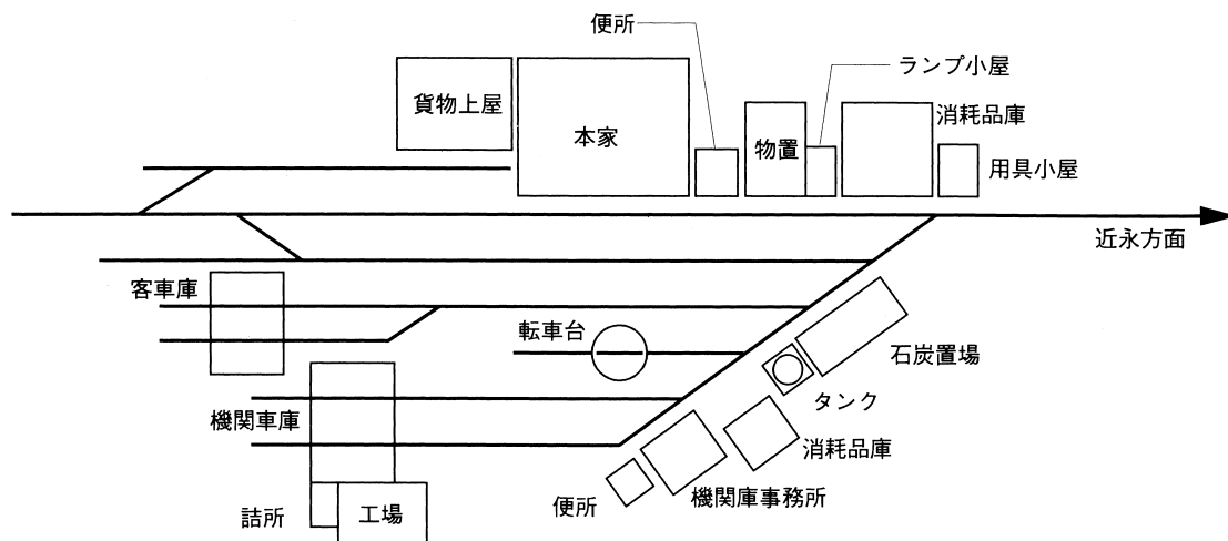
図2 初代宇和島駅構内配置図 「宇和島鉄道延長線設計図」を元に作成
