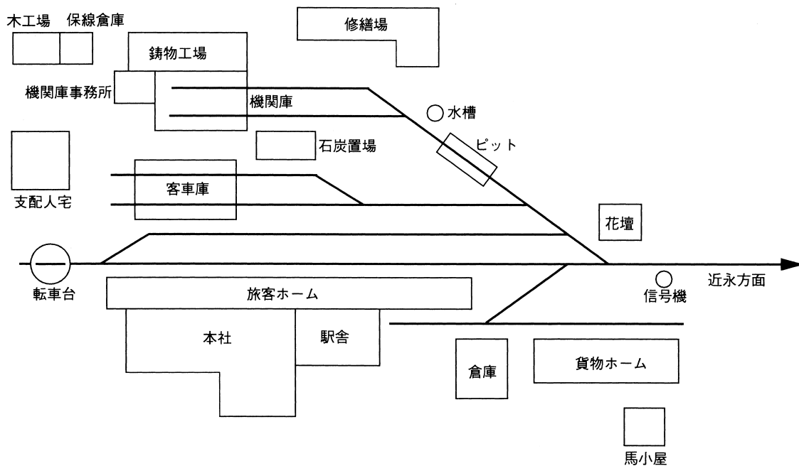
図3 2代目宇和島駅構内配置図 元宇和島機関区技工長尾崎正雄氏よりご教示いただいた内容を元に作成
