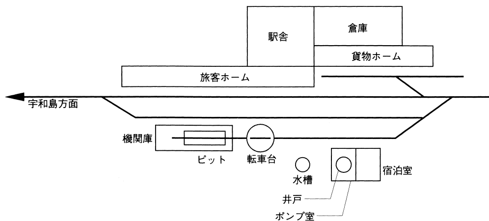
図4 吉野駅構内配置図 松野町柳野利男氏よりご教示いただいた内容を元に作成
