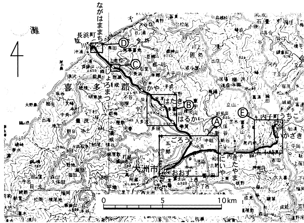
図5 愛媛鉄道路線図 駅名は白井茂信（1984 b）：国鉄狭軌軽便線15を参考にした 愛媛鉄道路線のうち現在の鉄道路線と位置が異なる部分に拡大図を付けた 国土地理院発行1/200,000地勢図「松山」より作成
