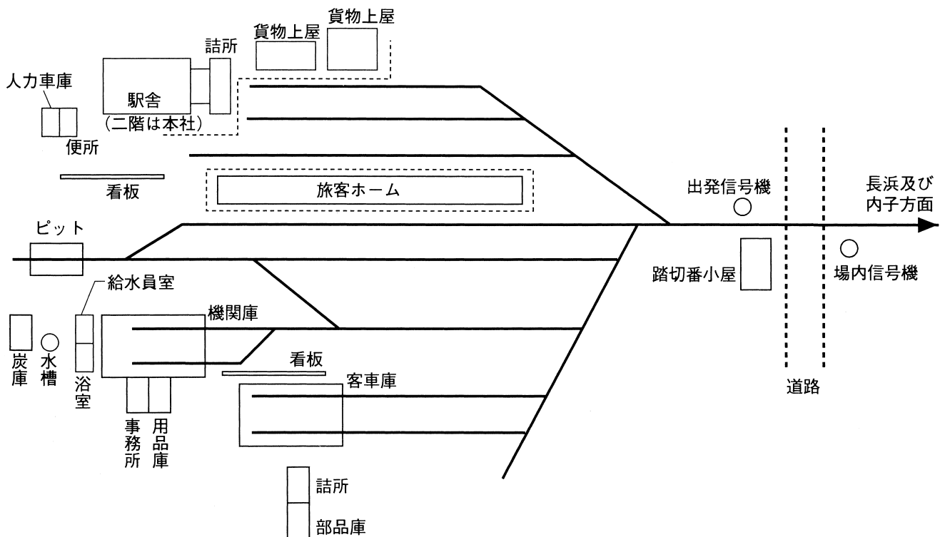
図6 旧大洲駅構内配置図 元愛媛鉄道職員 of 山本正氏・福山徳頼氏のご教示及び「愛媛鉄道国鉄移管記念写真帖」の写真をもとに作成
